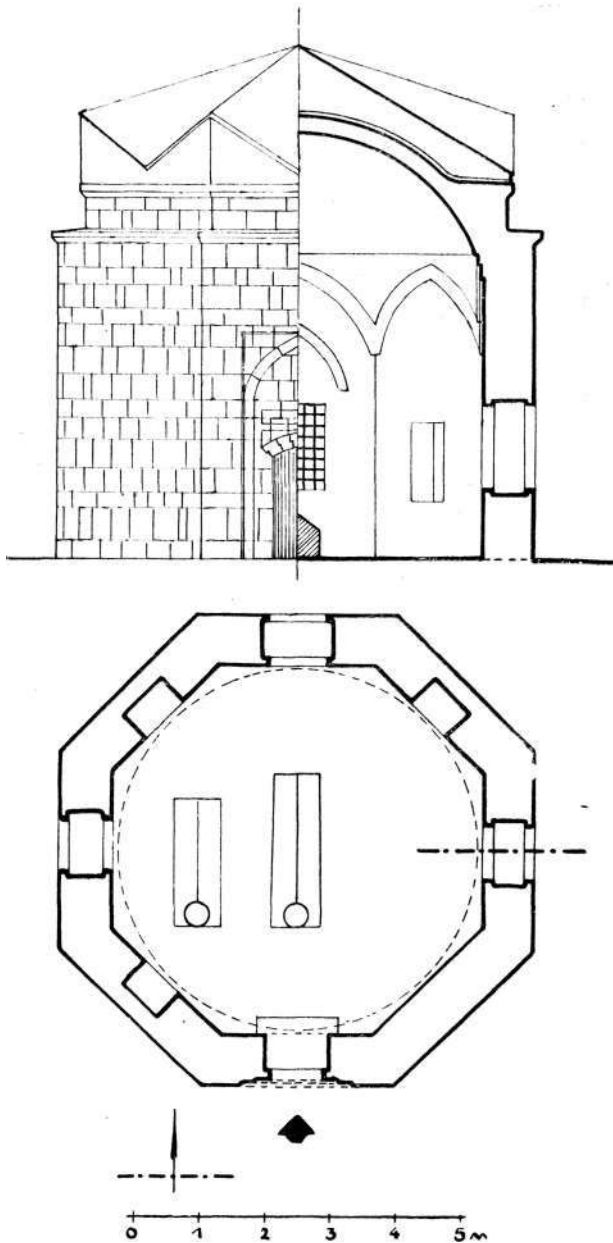
Halil-pašino turbe — presjek i tlocrt (Dž. Čelić — M. Go- loš, 1952)
