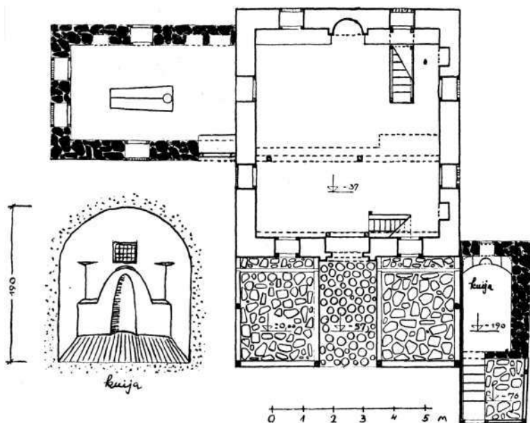
Behram-efendijina džamija s turbetom i kuijom — tlocrt (Dž. Čelić — M. Gološ, 1952)
