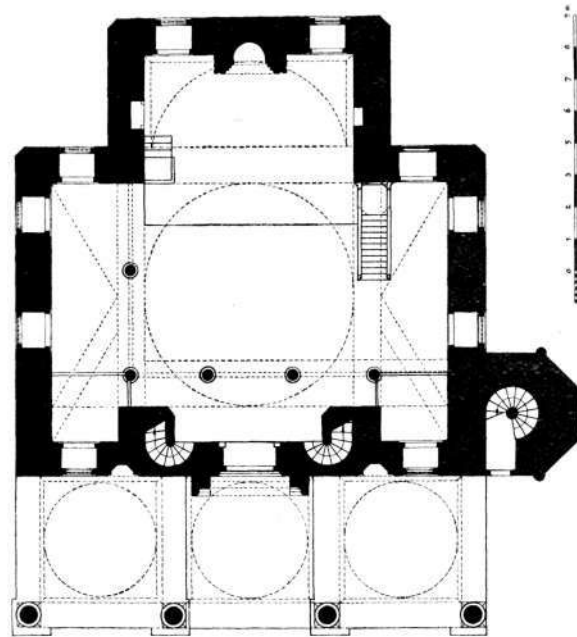
Džamija Ferhadija — tlocrt (arh. M. Fučić, 1952)
