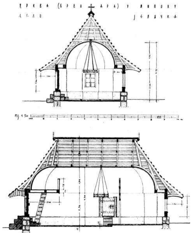
Crkva u Lipiku, selo Jelička, presjeci (ing. E. Dimitrijević, 1952)
