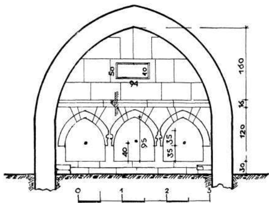
Česma u Klisu, presek a-a
