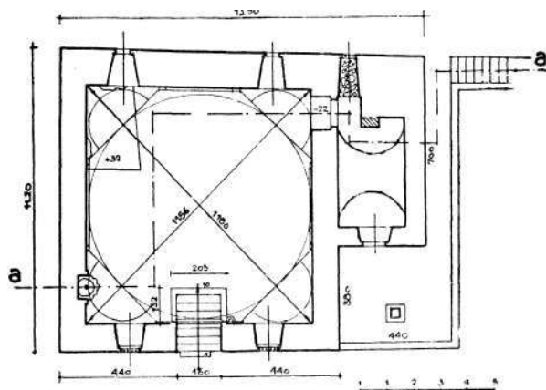
Džamija u Klisu, tlocrt
