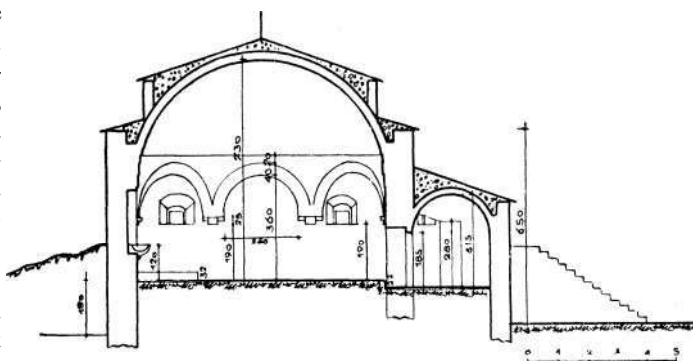
Džamija u Klisu, presek a- a
