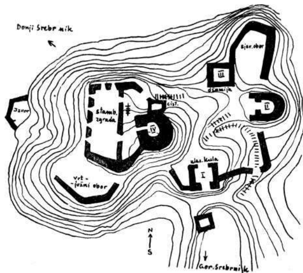
Sl. 7. Stari grad Srebrenik. Orijehtaciona skica. Grad još nije u cjelini snimljen, a ovaj kroki treba da pruži samo približnu sliku rasporeda građevina o kojima se govori u radu
