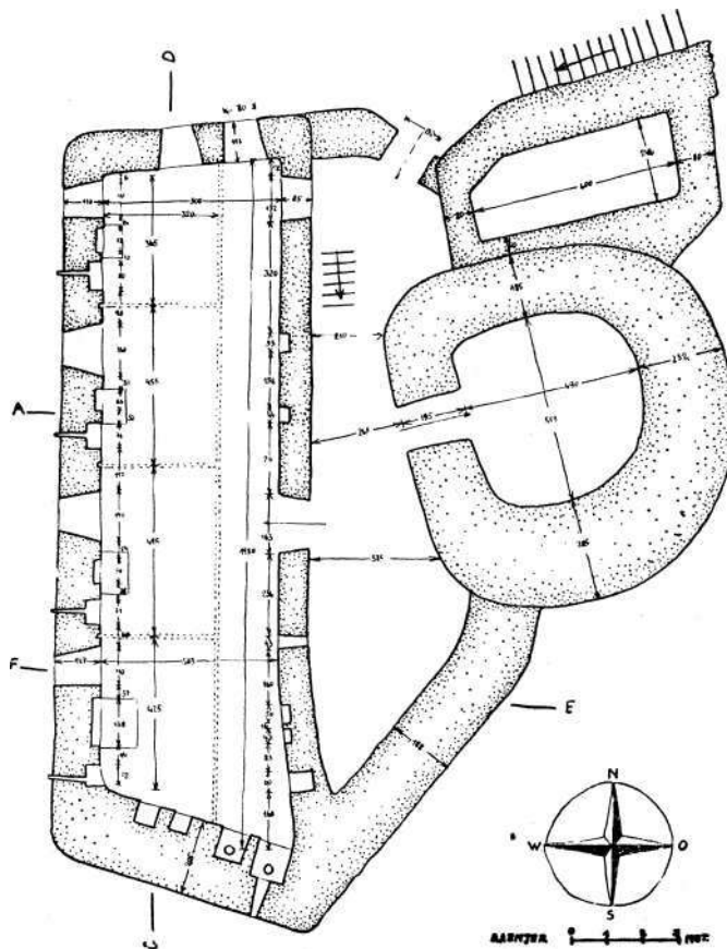
Sl. 9. Stari grad Srebrnik. Osnova stambene zgrade i glavne kule
