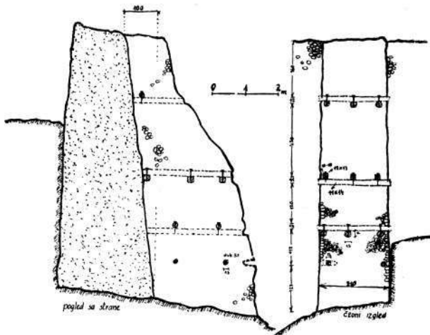
Sl. 8. Stari grad Ključ. Kontrafor na vanjskom zidu. Sistem zidanja pomoću drvene armature tipičan je za domaću arhitekturu Srednjeg vijeka i turskog doba. Zbog veličine, načina obrade i slaganja kamena u lice zida, nije, naime, dobiven statički dovoljno siguran oklop koji bi izdržao pritisak kaše od gašenog kreča i sitnog kamena, čime je popunjavana srž zida.
