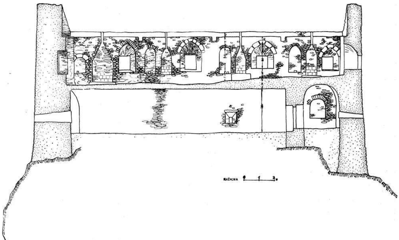
Sl. 11. Stari grad Srebrnik. Stambena zgrada, presjek C—D
