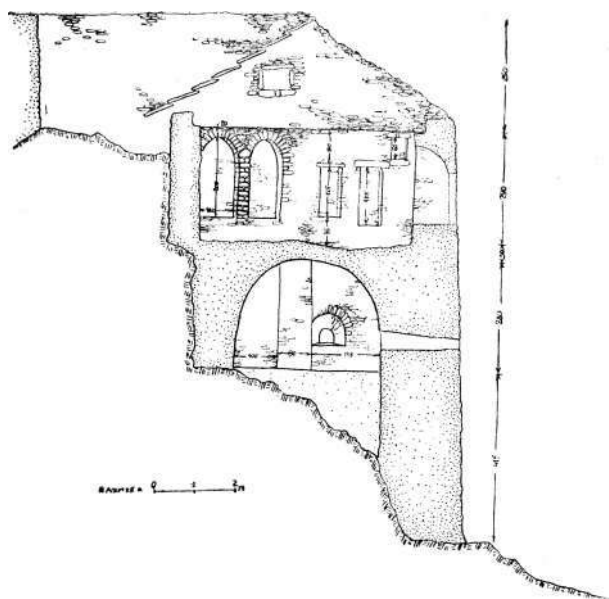
Sl. 12. Stari grad Srebrnik. Stambena zgrada, presjek E - F
