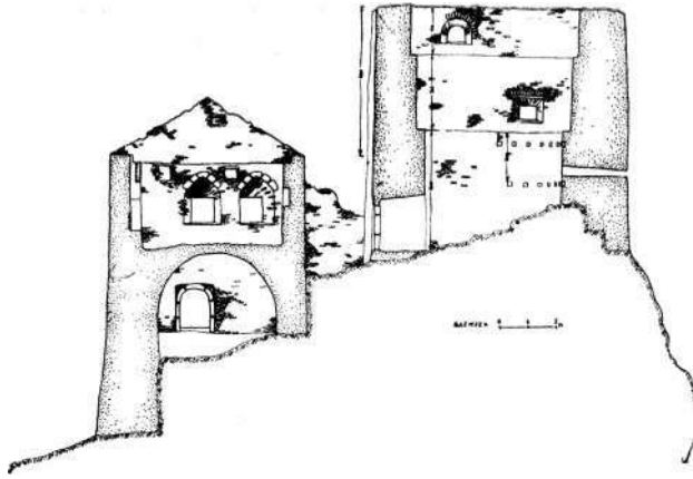
Sl. 10. Stari grad Srebrenik. Stambena zgrada i glavna kula, presjek A—B
