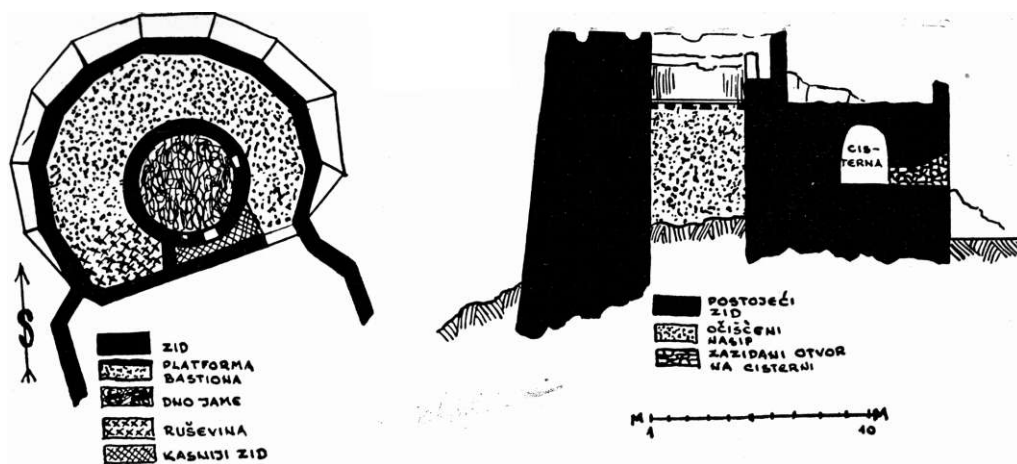
Sl. 3. Plan i presjek bastiona travničkog grada nakon otkrivanja šupljine u njemu
