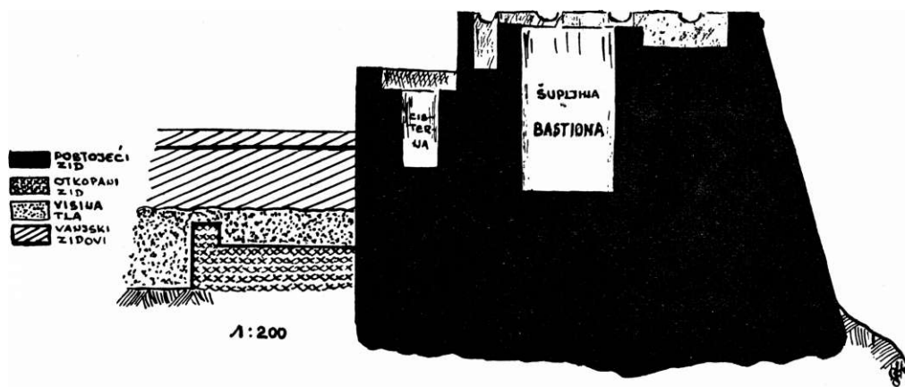
Sl. 4. Presjek bastiona i neposredne okolice na starom gradu u Travniku
